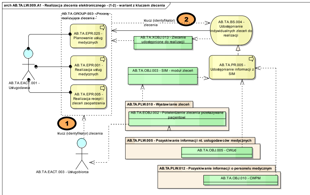
Rysunek 10 Realizacja zlecenia elektronicznego - wariant z kluczem zlecenia
